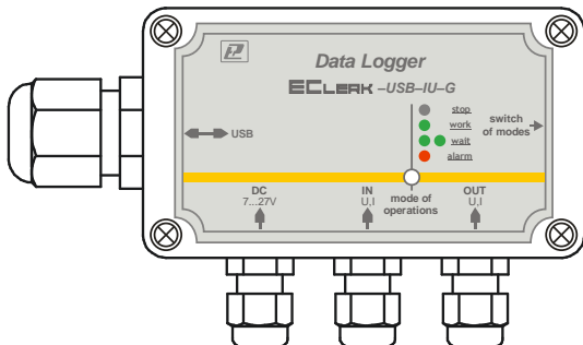
Рисунок 1– Внешний вид автономного регистратора унифицированных сигналов ECLERK®-USB-IU-G
