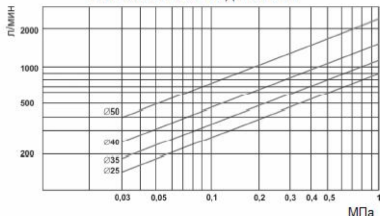
ДИАГРАММА ПРОПУСКНОЙ СПОСОБНОСТИ КЛАПАНОВ СЕРИИ 2W21 В ЗАВИСИМОСТИ ОТ ДАВЛЕНИЯ
